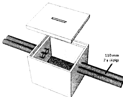
FIGURA 4. Características de las cajas de acceso (CA)
