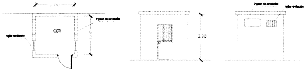
FIGURA 14. Cuarto común de telecomunicaciones superior (CCTS) - Perspectiva
