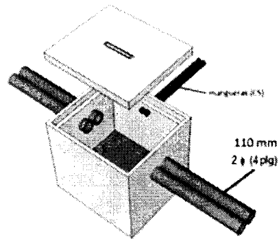
FIGURA 5. Caja de Paso (CP) - Perspectiva
