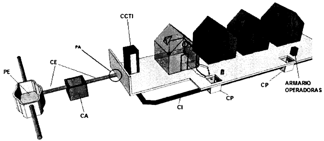
FIGURA 21. ICCT para viviendas unifamiliares - Perspectiva
