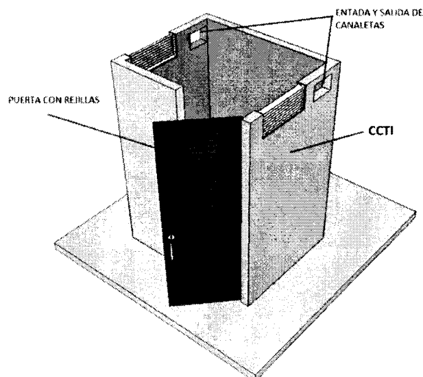
FIGURA 12. Cuarto común de telecomunicaciones inferior (CCTI) - Perspectiva
