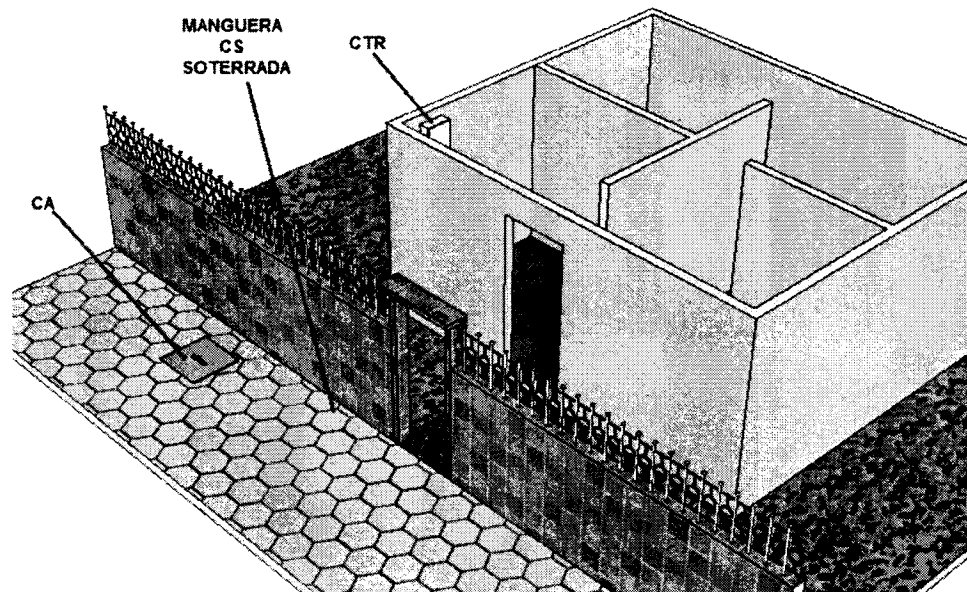
FIGURA 21. ICCT para viviendas unifamiliares - Perspectiva
