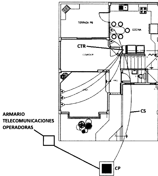
FIGURA 28. Distribución para condominios - Implantación
