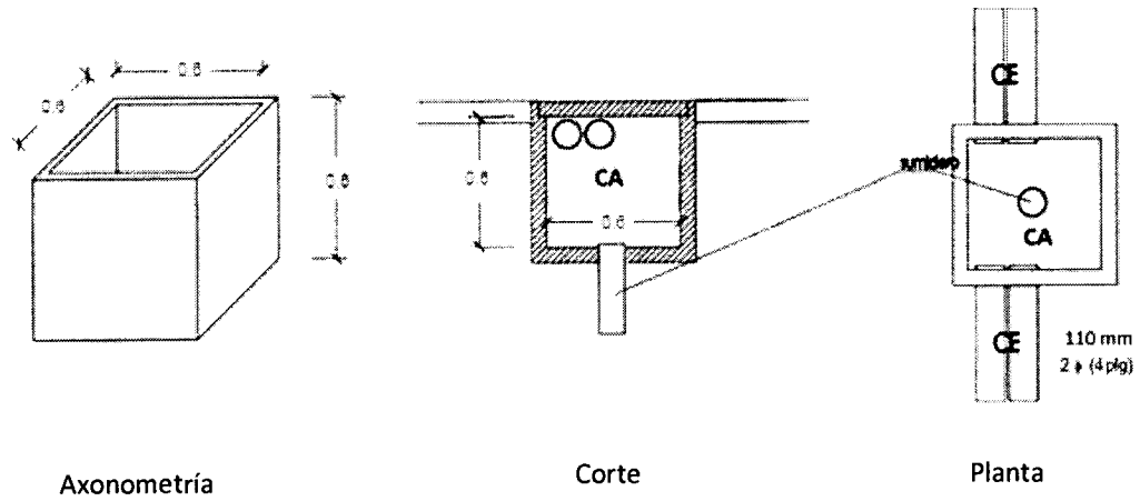
FIGURA 5. Caja de Paso (CP) - Perspectiva
