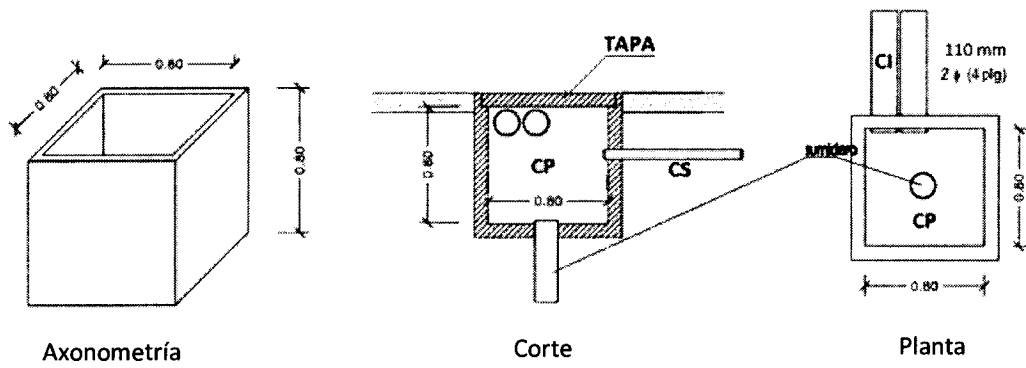
FIGURA 8. Canalización de Abonado (CU) - Perspectiva
