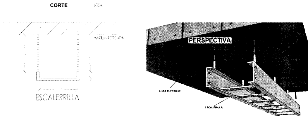
FIGURA 9. Canalización interna (CI)
