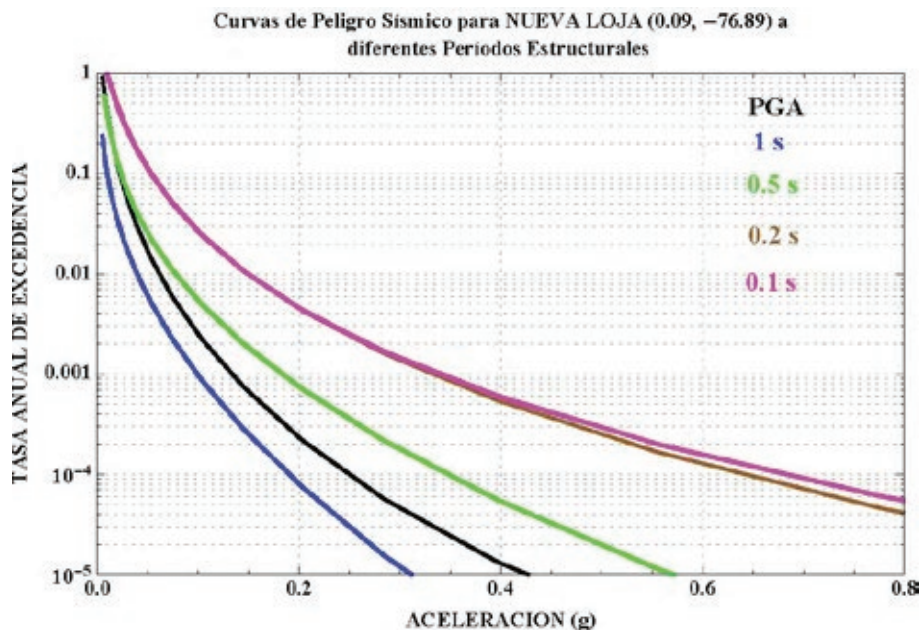
Figura 32: Curvas de peligro sísmico, Nueva Loja.
