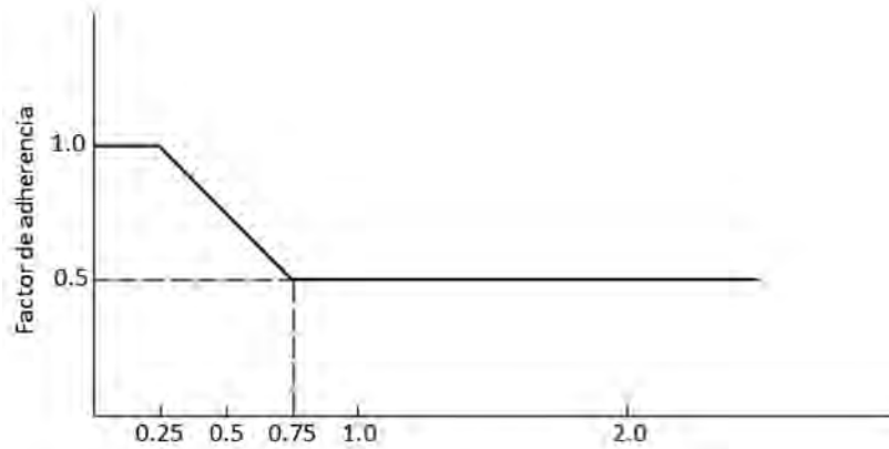
Figura 67: Factor \alpha recomendado por el USACE
