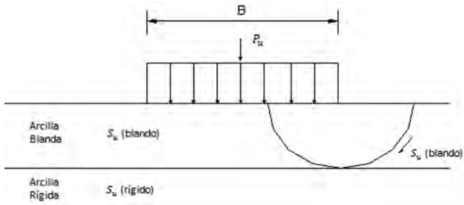
Figura 51: Mecanismo de Falla en Suelo Blando sobre Suelo Firme
