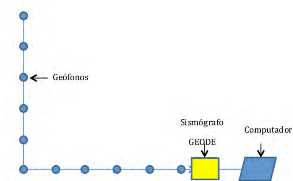
Figura 11: Arreglo geométrico contemplado para la adquisición de datos
