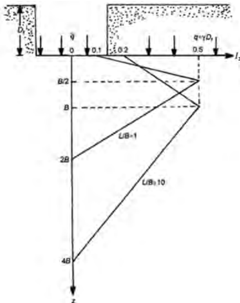
Figura 55: Variación de I_z versus z/B
