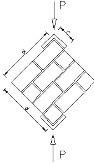
Figura 1: Carga en la dirección de la diagonal del murete
