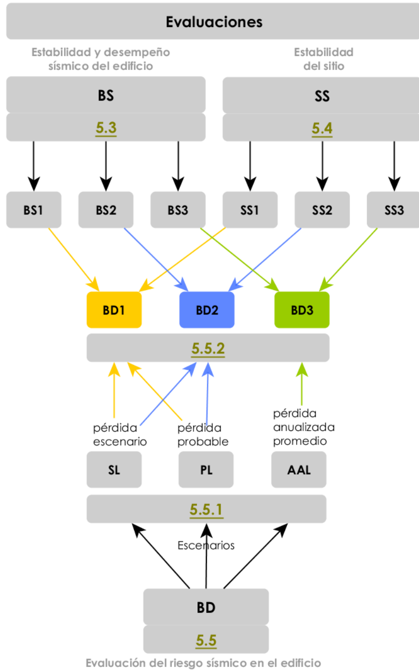
Figura 2: Esquema conceptual simplificado de evaluación sísmica de la NEC-SE-RE
